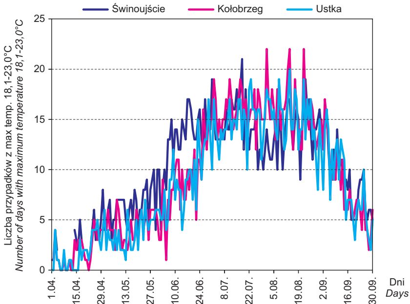
Ryc. 3. Przebieg ogólnej (w latach 1986-2013) liczby przypadków z maksymalną temperaturą powietrza 18,1-23,0 °C w okresie od kwietnia do września Course for the total number of days with maximum air temperature in the range 18.1-23.0 °C in the April-September period of the years 1986-2013
