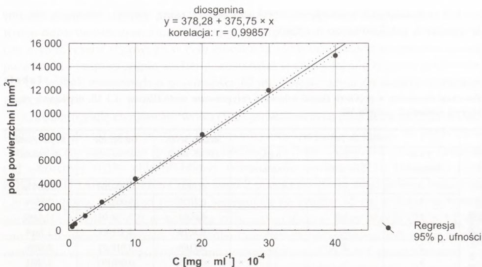
Rys. 1. Krzywa kalibracji.
