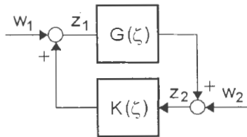
Rys. 1.2. Ilustracja problemu wewnętrznej stabilności.
