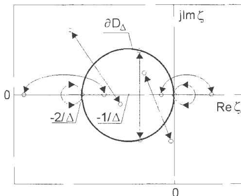
Rys 1.1. Ilustracja \delta -koniugacji.
