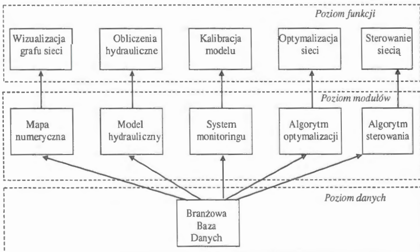
Rysunek 1. Struktura systemu wspomagania decyzji operatora sieci wodociągowej
