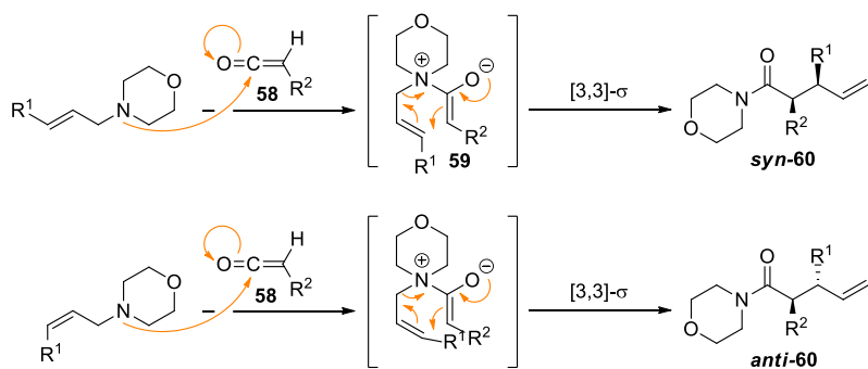
Schemat 48. Wariant przegrupowania aza -Claisena z ketenami.
