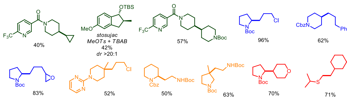
Schemat 110. Wybrane metody tworzenia wiązań \text{C}(\text{sp}^3)\text{-C}(\text{sp}^3) w warunkach fotoredoks.
