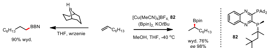
Schemat 71. Hydroborowanie okt-1-enu zgodne (po lewej) oraz niezgodne (po prawej) z regułą Markownikowa.
