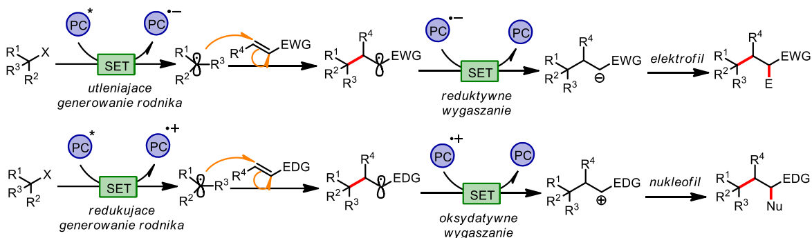
Schemat 106. Połączenie reaktywności rodnikowej i polarnej w warunkach fotoredukcji.
