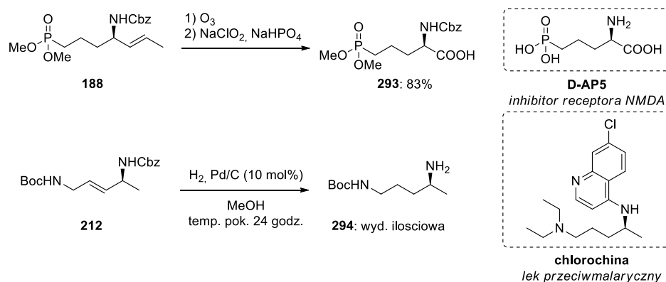
Schemat 142. Synteza prekursorów D-AP5 oraz chlorochiny.
