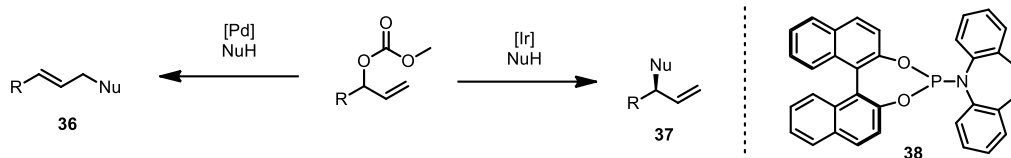
Schemat 28. Regiodywersja w reakcji Tsujiego-Trosta.
