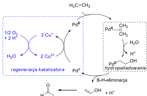
Schemat 86. Uproszczony mechanizm utlenienia Wackera.
