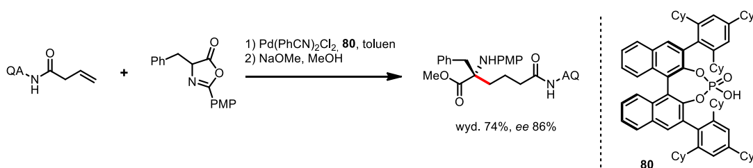
Schemat 67. Enancjoselektywne alkilowanie azlaktonów z wykorzystaniem nieaktywowanych alkenów.
