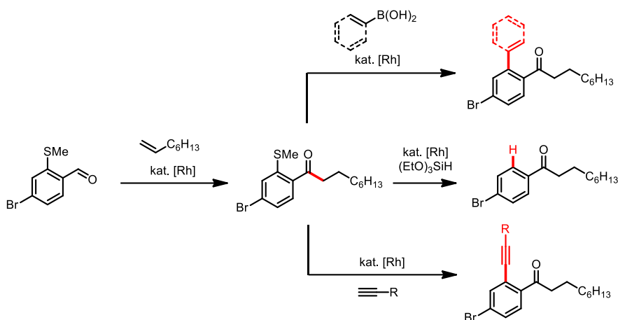
Schemat 73. Derywatywacja siarkowych produktów hydroacylowania.
