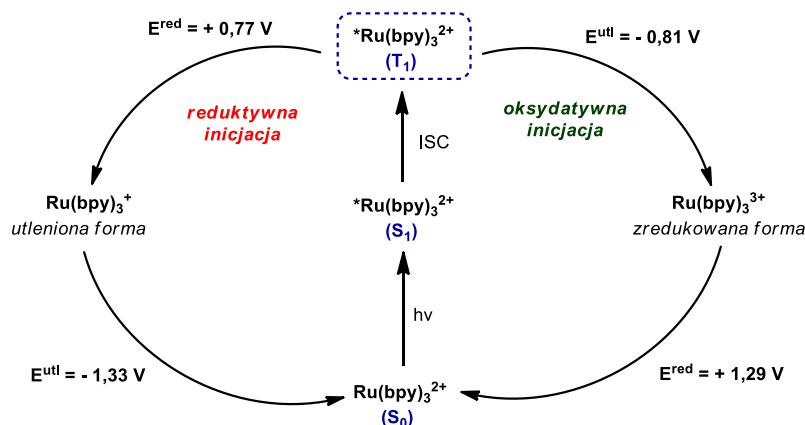
Schemat 92. Schemat możliwych reakcji redoks wzbudzonej formy katalizatora Ru(bpy)_3^{2+} .
