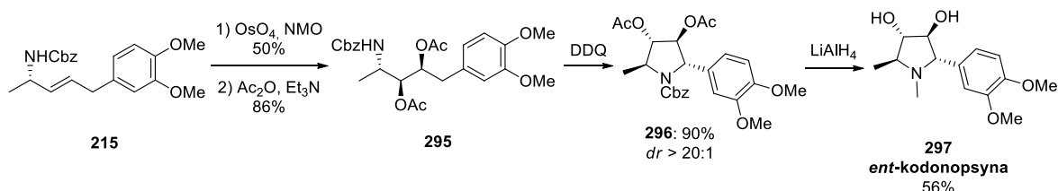
Schemat 143. Synteza enancjomeru alkaloidu kodonopsyny.
