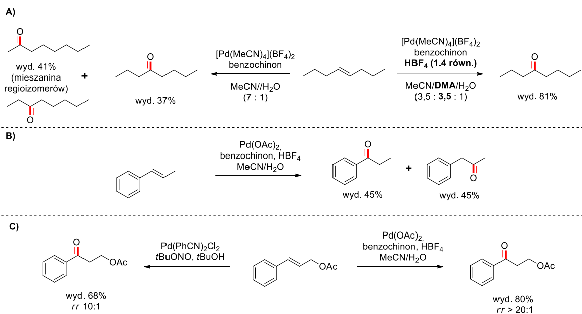
Schemat 89. Reakcja Wackera 1,2-dwupodstawionych olefin.
