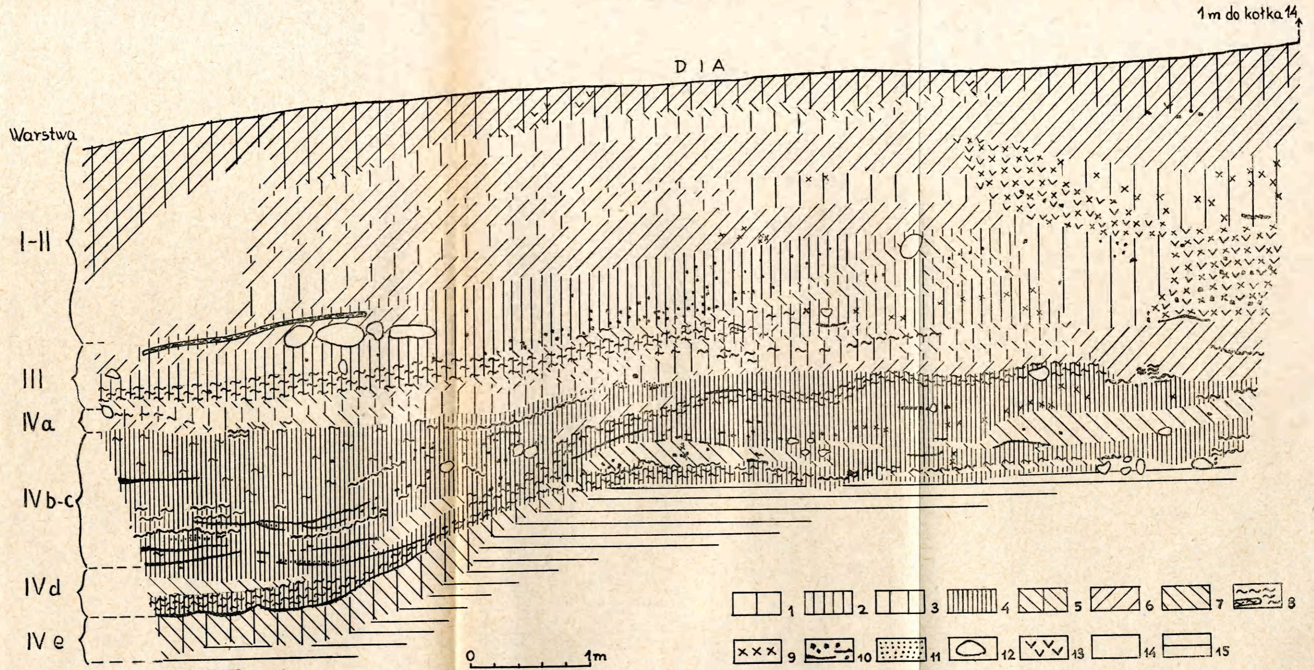
Ryc. 2. Czersk, pow. Piaseczno. Stanowisko 1 — „Zamek”. Profil zachodni wykopu 1 (ar 27, ćw. A, D):
