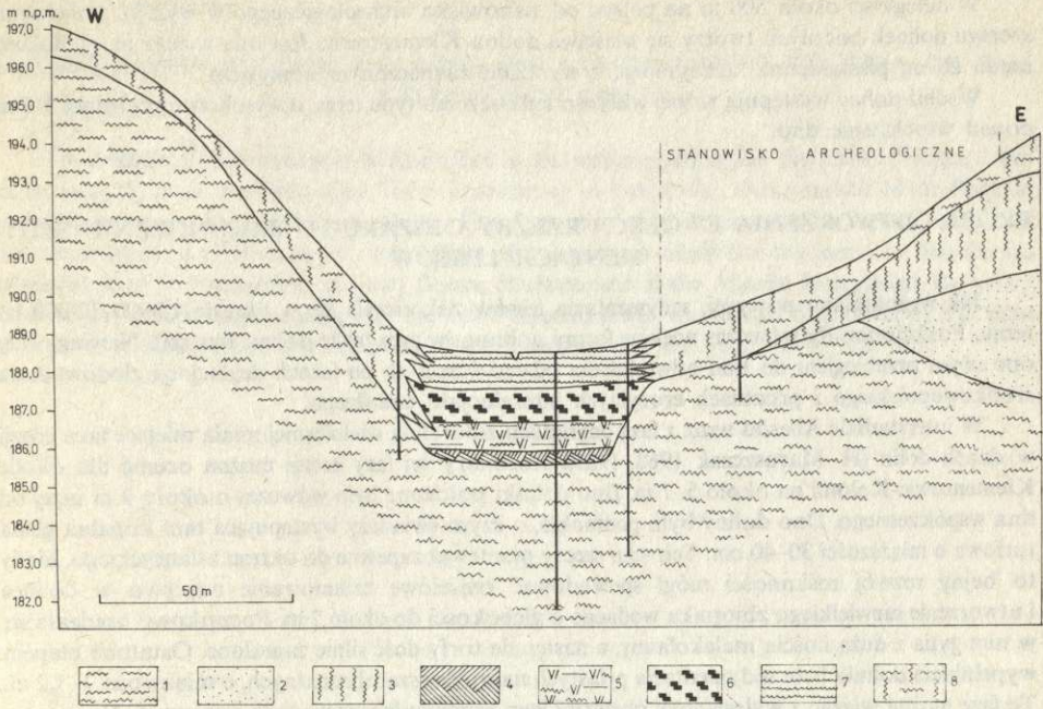
Ryc. 2. Przekrój geologiczny przez dolinę w okolicy Klementowice-Kolonii
