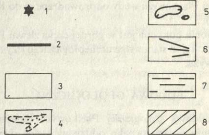
Ryc. 1. Szkic geomorfologiczny okolic Klementowice-Kolonii
