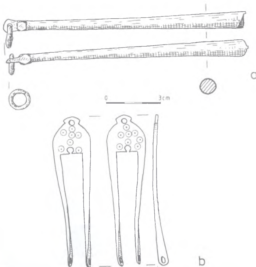
Ryc. 6. Fragmenty wag ze Szczecina: a – ramię wagi typu III z kwartału 6., XIII/XIV w. (rys. H. Bona); b – imadelko wagi z kwartału 6., 1.-2. ćw. XIII w. (rys. H. Bona)
