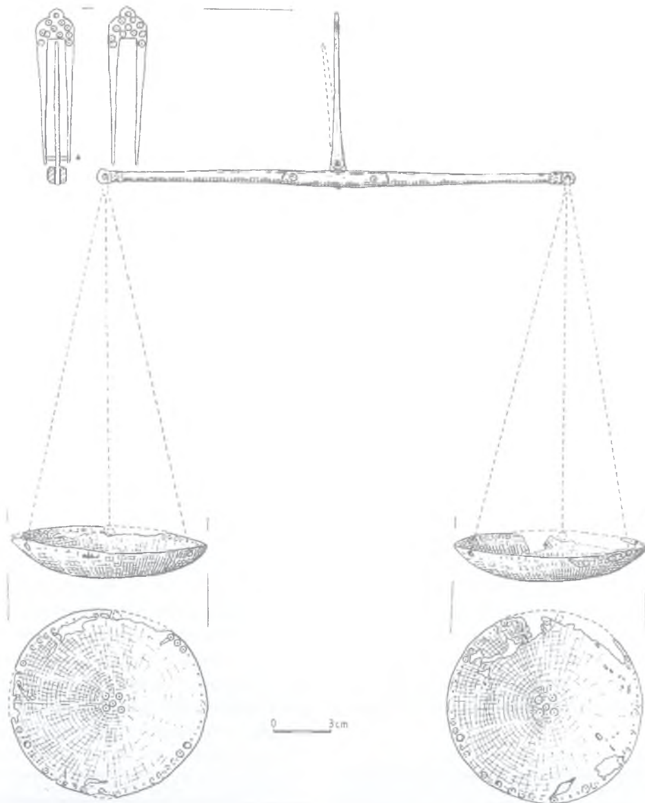
Ryc. 4. Waga typu II z kwartału 6., pocz. XIII w. (rys. H. Bona) Abb. 4. Waage vom Typ II aus dem Quartier 6, Beginn des 13. Jh. (gez. von H. Bona)
