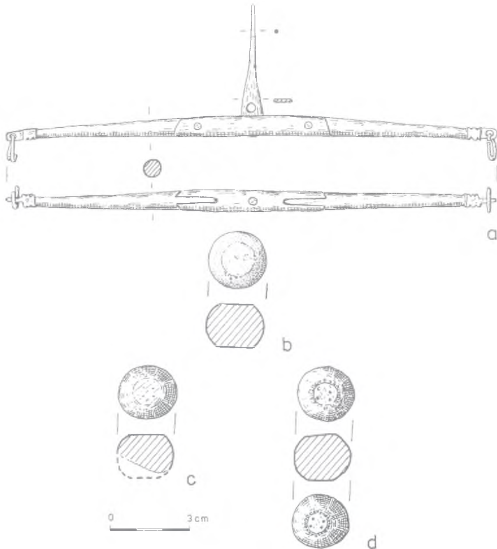
Ryc. 5. Przybory kupieckie ze Szczecina: a – waga typu IIb ze Szczecina, bez lokalizacji, XII w. (rys. H. Bona); b – odważnik z kwartału 6., poł. XI w. (rys. K. Kowalski); c-d – odważniki z kwartału 5., 2 poł. XII w. (rys. H. Bona) Abb. 5. Kaufmännisches Zubehör aus Szczecin: a – Waage vom Typ IIb aus Szczecin, ohne Fundortangaben, 12. Jh. (gez. von H. Bona); b – Wägestück aus dem Quartier 6, Mitte des 11. Jh. (gez. von K. Kowalski); c-d – Wägestücke aus dem Quartier 5, 2. Hälfte des 12. Jh. (gez. von H. Bona)
