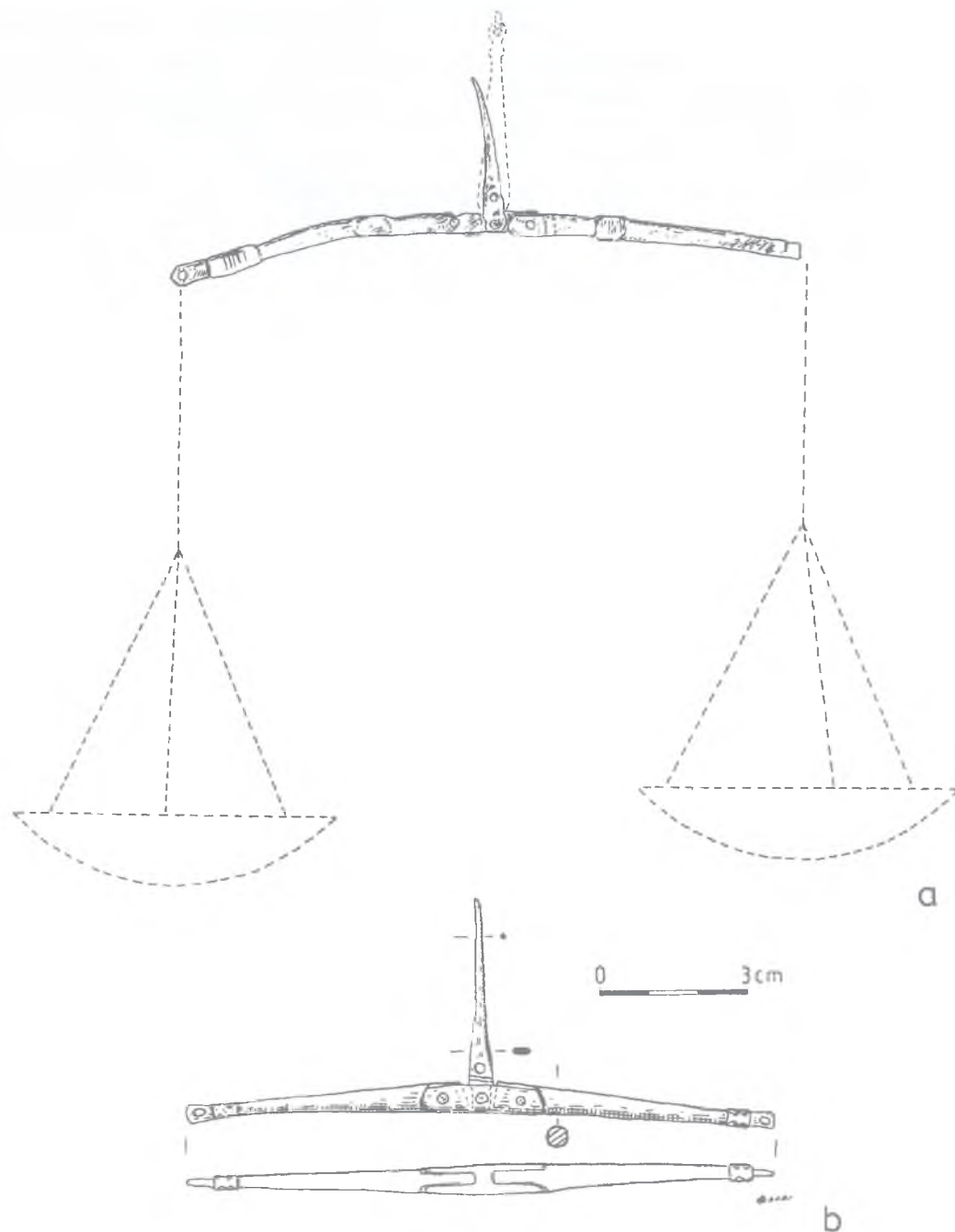
Ryc. 3. Wagi ze Szczecina: a – waga typu Ic ze Wzgórza Zamkowego, 1 poł. XII w. (rys. H. Bona);
