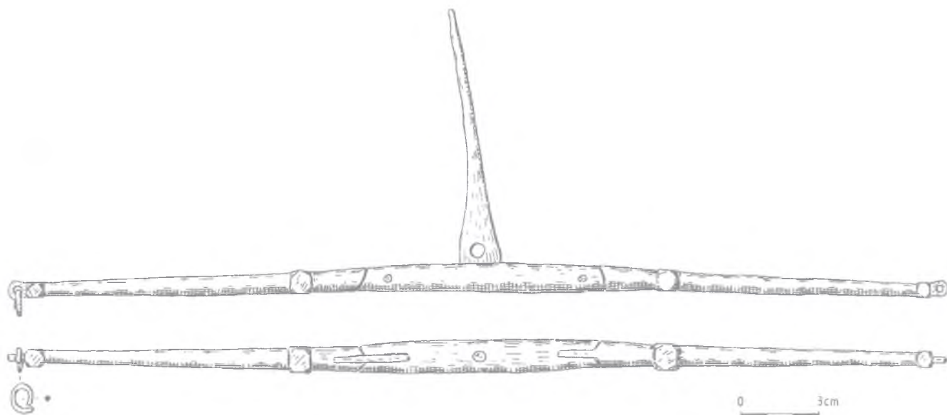
Ryc. 7. Waga składana typu III z kwartału 6., XIII/XIV w. (rys. H. Bona) Abb. 7. Klappwaage vom Typ III aus dem Quartier 6, 13./14. Jh. (gez. von H. Bona)
