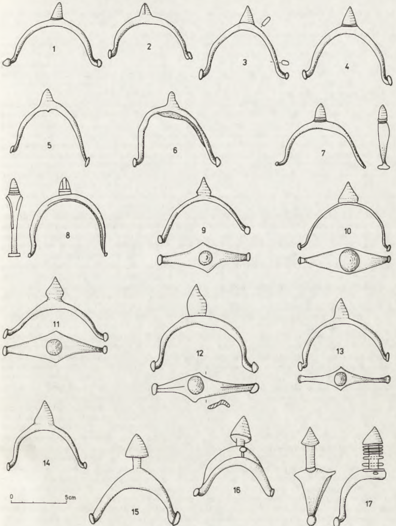
Ryc. 13. Ostrogi kabłakowe podgrupy F - Bügelsporen der Untergruppe F: Typ F1 (1-4 - Variante F1a, 5, 6 - Variante F1b), Typ F2 (7, 8), Typ F3 (9-12 - Variante F3a, 13, 14 - Variante F3b), Typ F4 (15-17)
