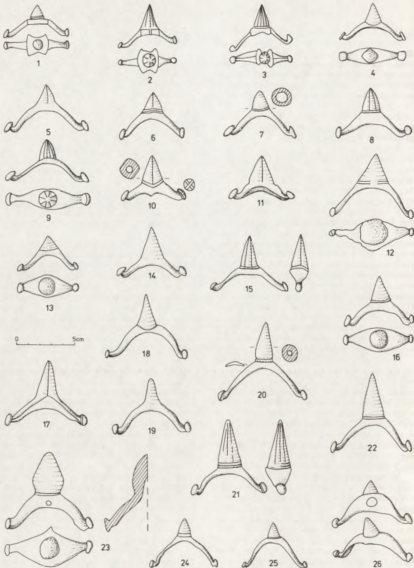
Ryc. 11. Ostrogi kabłąkowe podgrupy E - Bügelsporen der Untergruppe E: Typ E1 (1-3), Typ E2 (4-9), Typ E3 (10, 11), Typ E4 (12, 13), Typ E5 (14-17 - Variante E5a, 18, 19 - Variante E5b), Typ E6 (20-22), typ E7 (23), typ E8 (24, 25 - Variante E8a, 26 - Variante E8b)
