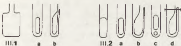
Ryc. 4. Warianty zaczepu zachodnich ostróg oczkowych – Befestigungsvarianten der westlichen Ösensporen
