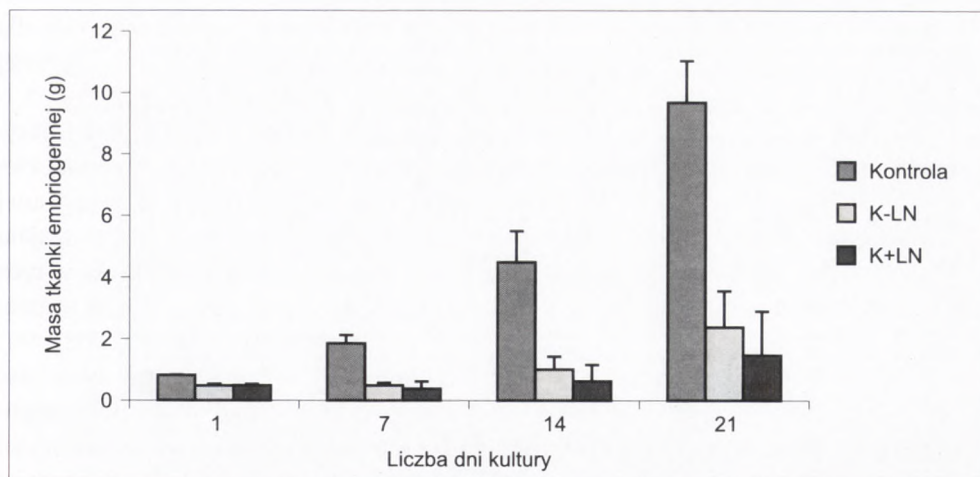
Rys. 3. Wzrost (g świeżej masy) tkanki embriogenicnej Picea omorika , rozmrożonej z ciekłego azotu w trakcie 21-dniowej kultury na pożywce namnażającej \frac{1}{2} LM. Kontrola – tkanka nie mrożona, K-LN-1 i K+LN jak na rys. 2.
