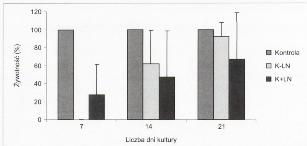
Rys. 2. Żywotność (%) tkanki embriogennej w trakcie 21-dniowej kultury po rozmrożeniu z ciekłego azotu. Kontrola – tkanka nie mrożona, K-LN-1 i K+LN jak na rys. 1.
