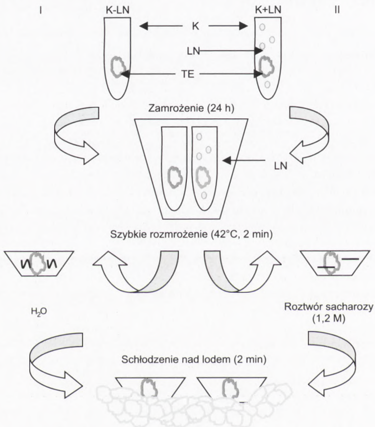
Rys. 1. Schemat zamrażania i rozmrażania tkanki embriogennej świerka serbskiego z ciekłego azotu dwoma sposobami: I K-LN – wariant mrożenia tkanki bez dodatku ciekłego azotu do krioprobówki; II K+LN – wariant mrożenia tkanki z dodatkiem ciekłego azotu do krioprobówki; K – krioprobówka, LN – ciekły azot, TE – tkanka embriogenna.
