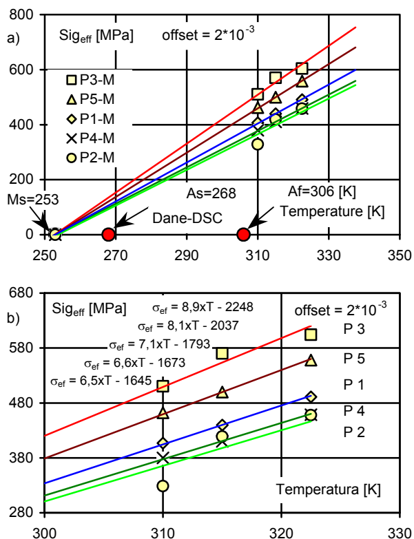
Rys. 5.9 a) Relacje Clausiusa-Clapeyrona – CC dla przemiany A→M w zakresie pseudosprężystego zachowania stopu NiTi i przemiany monoklinicznej. Punktami zaznaczono wartości doświadczalne. Linie stanowią interpolacje wyznaczone metodą najmniejszych kwadratów przy ich ekstrapolacji do punktu ( \sigma_{eff} = 0, T = 253 K ), tj. temperatury początku przemiany martenzytycznej w stanie beznaprężeniowym. b) Położenie punktów doświadczalnych relacji Clausiusa-Clapeyrona w zbliżeniu oraz wartości doświadczalne nachyleń linii CC wyznaczonych interpolacyjnie metodą najmniejszych kwadratów.
