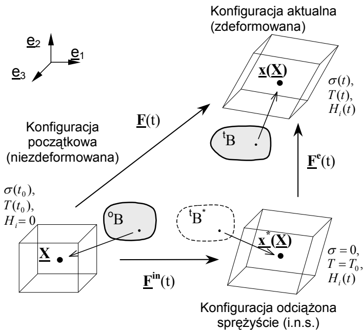
Rys. 7.1 Kinematyka skończonych deformacji.
