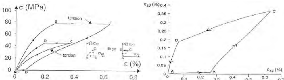
Rys. 3.8 Test dwuosiowego nieproporcjonalnego rozciągania-skręcania próbek polikrystalicznej CuZnAl. Za Roquedą i innymi [71].
