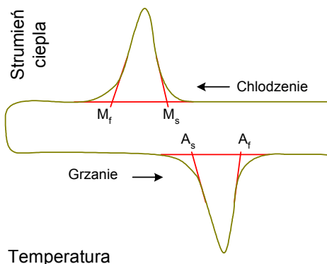
Rys. 2.1 Typowy wynik testu kalorymetrii różnicowej (DSC) dla materiału podlegającego martenzytycznej przemianie fazowej, w szczególności dla stopu z pamięcią kształtu.
