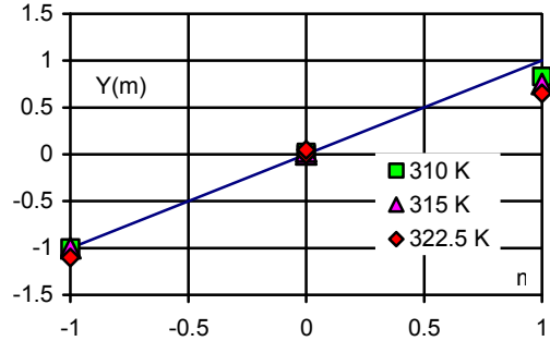
Rys. 5.11 Funkcja Y(m) - kryterium weryfikacji izotropii niesprężystej.
