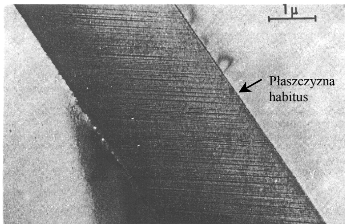
Rys. 2.4 Zdjęcie płytki martenzytycznej w stopie Fe30%Ni0.4%C ujawniające jej substrukturę bliźniaczą, uzyskane metodą elektronicznej mikroskopii transmisyjnej. Za Maki i Waymanem [52].
