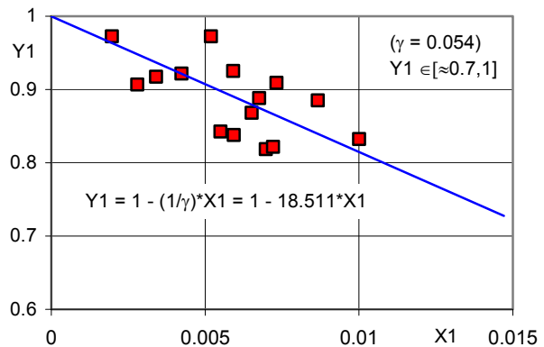
Rys. 5.13 Wyznaczenie amplitudy pływnięcia pseudosprężystego \gamma . Punkty oznaczają dane doświadczalne. Linia trendu została wyznaczona metodą najmniejszych kwadratów.
