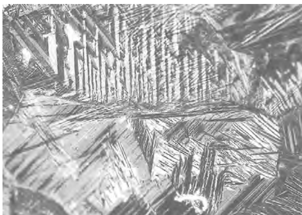
Rys. 2.7 Samoakomoduująca się mikrostruktura fazy martenzytycznej indukowanej temperaturą w polikryształe CuAlNiMn przy zerowym naprężeniu zewnętrznym. Za Leclercqiem i LExcellentem [37].
