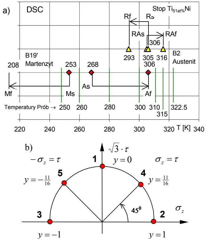
Rys. 5.1 a) Temperatury izotermicznych prób mechanicznych w porównaniu z charakterystycznymi temperaturami przemian fazowych – DSC. b) Schemat programu obciążeń mechanicznych.
