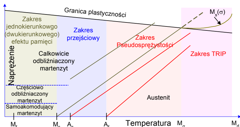
Rys. 2.9 Schematyczna mapa zakresu parametrów stanu w jakich dominującą rolę odgrywają różne efekty pamięci kształtu.
