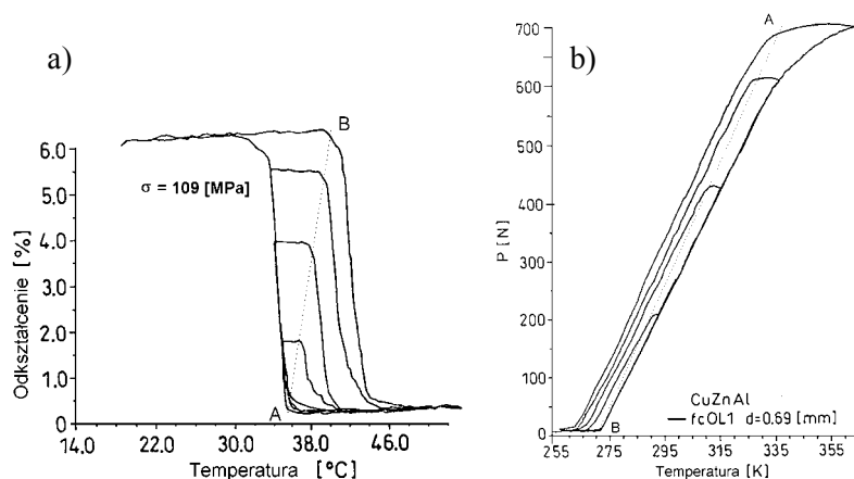
Rys. 3.3 a) Graniczna i wewnętrzne pętle histerezy we współrzędnych odkształcenie-temperatura dla próbki CuZnAl wynikające z obciążania próbki utrzymywanej pod stałym naprężeniem cyklami temperaturowymi – izostatyczne cykle temperaturowe. b) Zjawiska nawrotu (odzysku) siły występujące na skutek ogrzewania próbki CuZnAl. Za Huo i Müllerem [31].
