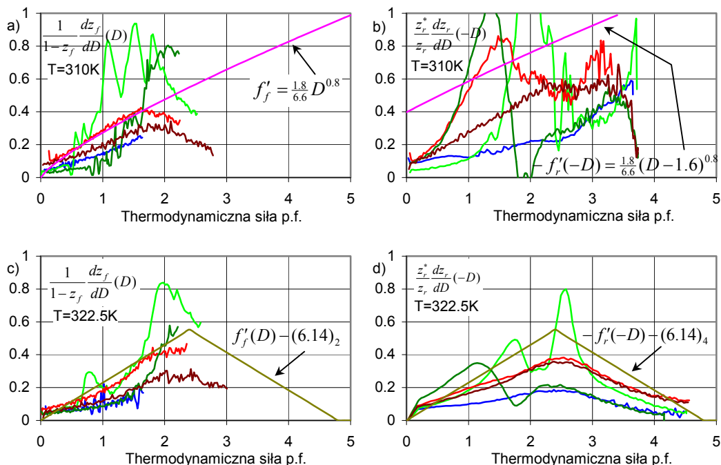
Rys. 6.9 Doświadczalne przebiegi prędkości właściwych dla pełnych przemian wprost i cząstkowych przemian odwrotnych w temperaturach 310K i 322.5K. Na wykresach 6.9a), 6.9b) wykreślono także dla porównania przebiegi prędkości właściwej przewidywanej przez model kinetyki R-L, por. (6.13) 1 , dla przemiany pełnej wprost i cząstkowej przemiany odwrotnej przy z^* = 0.4 . Na wykresach 6.9c), 6.9d) wykreślono dla porównania przebiegi prędkości właściwej przewidywanej przez model kinetyki proponowany w niniejszej pracy, por. (6.14).
