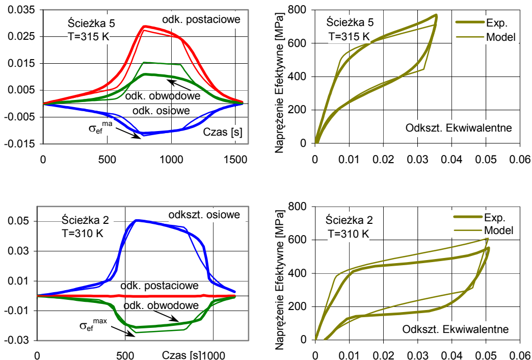
Rys. 5.14 Porównanie rzeczywistych przebiegów czasowych składowych \varepsilon_z(t) , \varepsilon_\theta(t) , \varepsilon_{z\theta}(t) tensora całkowitego odkształcenia z przebiegami przewidywanymi modelem R_L oraz porównanie rzeczywistych przebiegów \sigma_{ef} - \varepsilon_{eq} z przebiegami modelowymi w przypadku a) Próba w temperaturze 315 K, ścieżka 5. b) Próba w temperaturze 310K, ścieżka 2.
