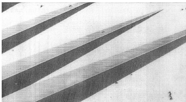
Rys. 2.5 Płytki martenzytyczne w kształcie klinów z widoczną wewnętrzną strukturą bliźniaczą. Za Otsuką i Waymanem [52].
