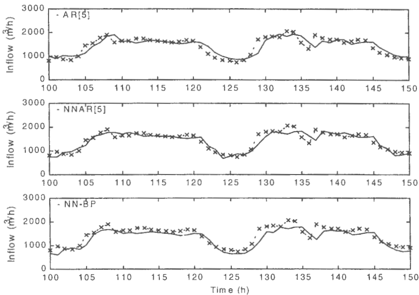
Rys. 4. Wyniki modelowania dla modelu ARMA (wykres górny) i dla dwóch modeli neuronowych (linia przerywana oznacza pomiary).
