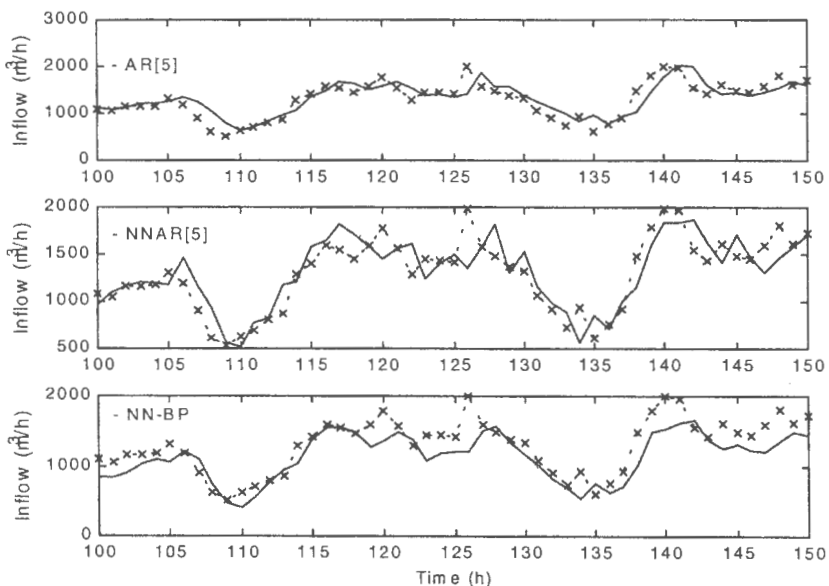
Rys. 6. Wyniki trenowania sieci neuronowej dla dwóch parametrów sterujących (punkty - pomiary, linia ciągła - model)
