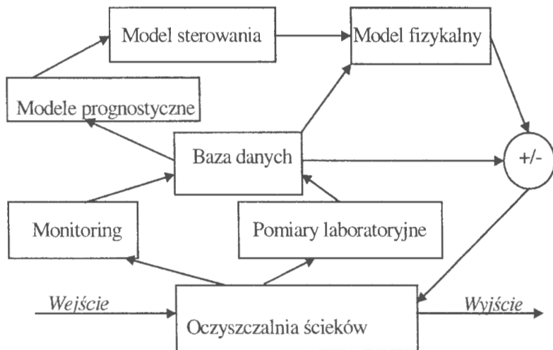
Rys. 3. Schemat systemu komputerowego dla oczyszczalni ścieków.
