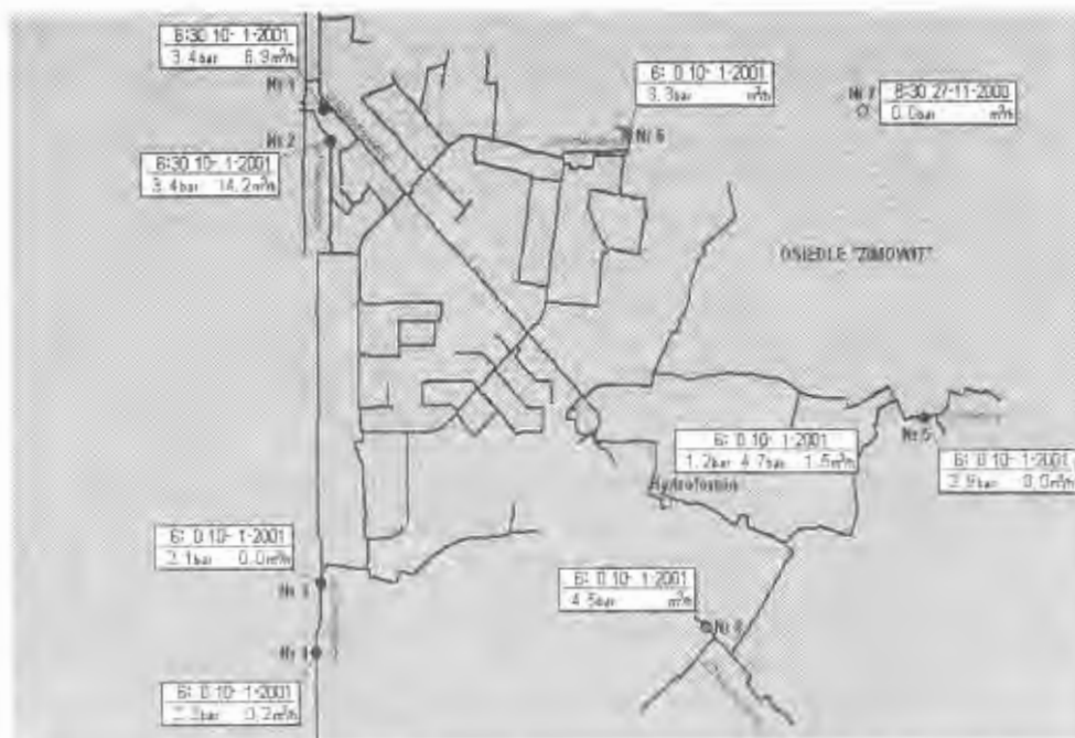
Rys. 1. Fragment sieci wodociągowej Rzeszowa objętej pilotowym systemem wspomaganie decyzji i systemem monitoringu.
