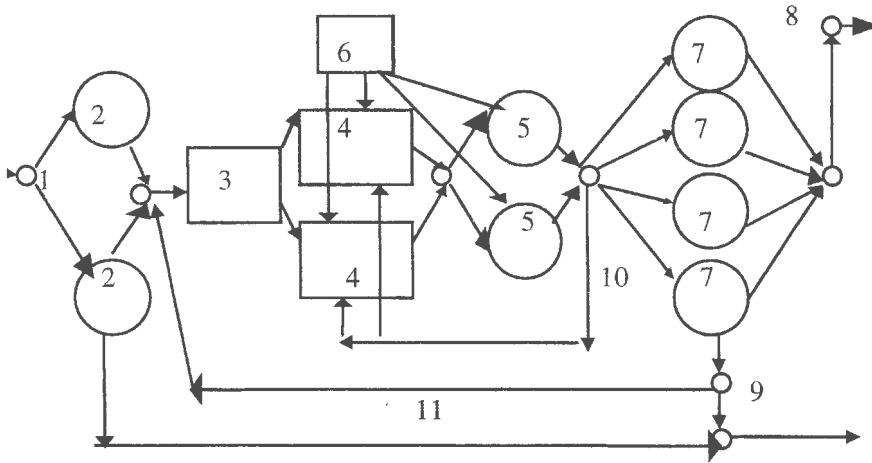
Rys. 2. Schemat oczyszczalni ścieków.
