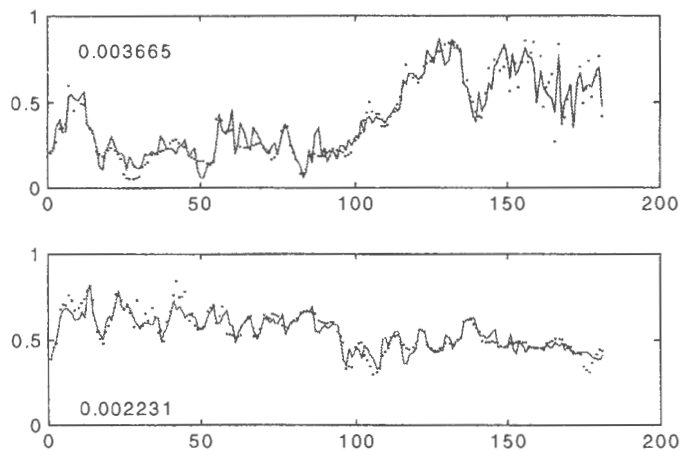
Rys. 5. Wyniki prognozowania dla modelu ARMA (wykres górny) i dla dwóch modeli neuronowych.
