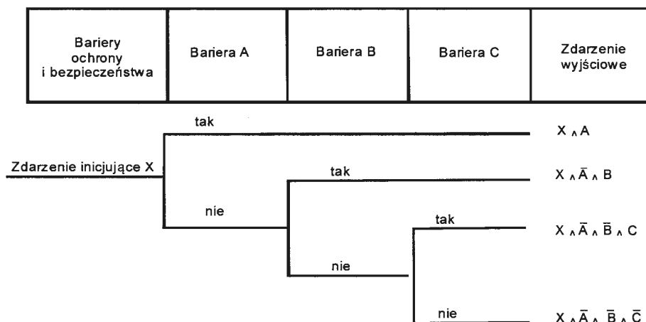
Rys. 17. Rozwój zdarzenia X względem bariery C.
