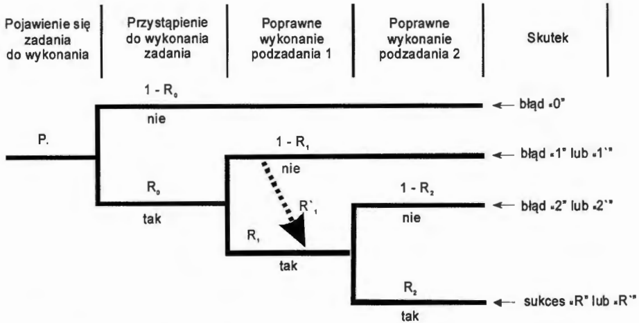
Rys. 18. Drzewo zdarzeń dla wykonania zadania przez operatora z możliwością poprawy popełnionego błędu.
