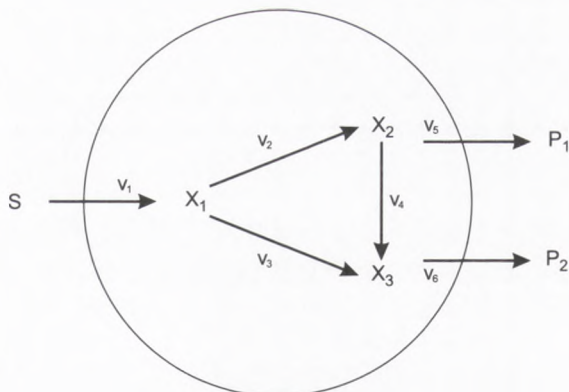
Rys. 3. Schemat prostej sieci metabolicznej.
