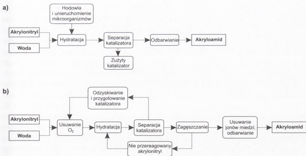
Rys. 2. Schemat produkcji akryloamidu metodą biotechnologiczną (a) i za pomocą konwencjonalnej syntezy chemicznej (b), rys. wg (2).
