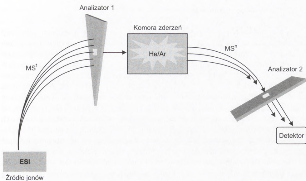
Rys. 2. Schemat przedstawiający zasadę działania tandemowego spektrometru mas wykorzystującego kolizyjnie indukowaną dysocjację jonów (CID MS/MS, ang. collision induced dissociation tandem mass spectrometry ).
