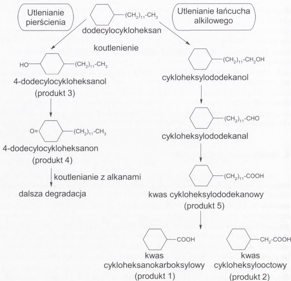
Rys. 3. Biodegradacja dodecylcycloheksanu (28,29).
