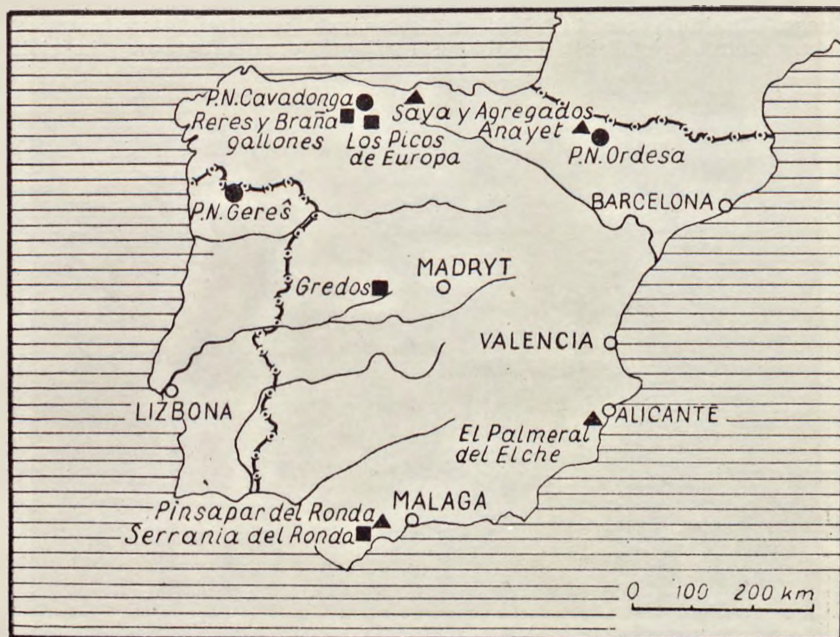
Ryc. 1. Rozmieszczenie obszarów objętych ochroną w Hiszpanii i Portugalii: 1 — parki narodowe, 2 — rezerwy, 3 — chronione tereny państwowe „Cotos nacionales”. (Według atlasu rezerwatów przyrodniczych świata — Derniers refuges )
