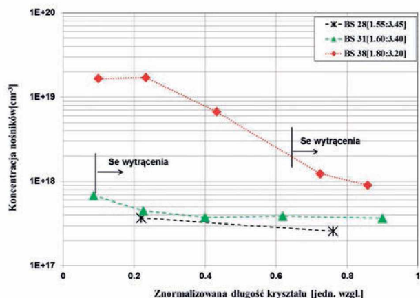
Rys. 16. Rozkład koncentracji nośników wzdluz kryształów \text{Bi}_2\text{Se}_3 wzrastających z cieczy o różnym nadmiarze selenu. Fig. 16. Carrier concentration distribution along crystals grown from the melt with a different selenium excess.
