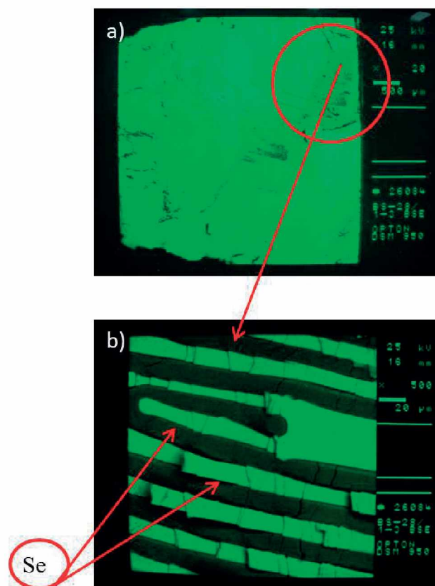
Rys. 24. Obraz SEM w brzegowej części na końcu monokryształu BS nr 28 a) x 20, b) x 500.
