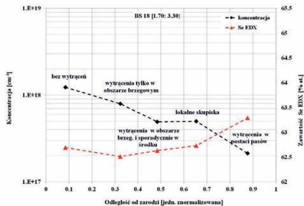
Rys. 18. Rozkład koncentracji nośników i zawartości selenu wzdluz kryształu BS – 18. Fig. 18. Carrier concentration and selenium content distribution along the BS – 18 crystal.
