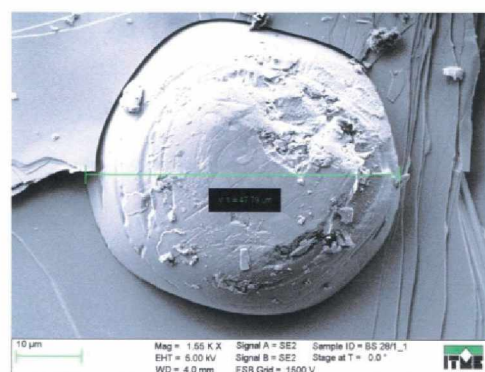
Rys. 23. Obraz SEM precypitatu Se wewnątrz bloków kwintetów kryształu \text{Bi}_2\text{Se}_3 nr 28 o składzie Bi:Se [1.55:3.45].
