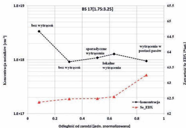
Rys. 17. Rozkład koncentracji nośników i zawartości selenu wzdluz kryształu BS – 17. Fig. 17. Carrier concentration and selenium content distribution along the BS – 17 crystal.
