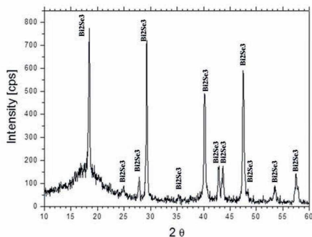
Rys. 25. Dyfraktogram z obszaru \sim 0,7 długości kryształu BS-18. Fig. 25. X-ray diffractogram of the BS-18 crystal at \sim 0.7 of its length.
