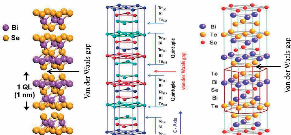
Rys. 2. Struktura warstwowa kryształów \text{Bi}_2\text{Se}_3 , \text{Bi}_2\text{Te}_3 i \text{Bi}_2\text{Te}_2\text{Se} [2 - 4].
