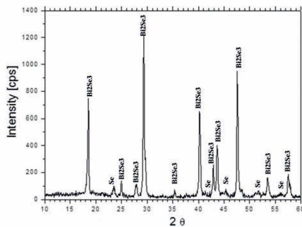
Rys. 26. Dyfraktogram z obszaru \sim 0,9 długości kryształu BS-18. Fig. 26. X-ray diffractogram of the BS-18 crystal at \sim 0.9 of its length.
