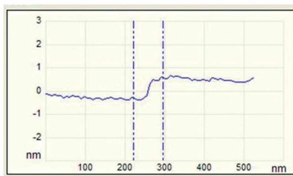
Rys. 11. Obraz AFM powierzchni płytki eksfoliowanej z kryształu \text{Bi}_2\text{Se}_3 z widocznym uskokiem odpowiadającym grubości jednej warstwy kwintetowej (ok. 1 nm) [11].
