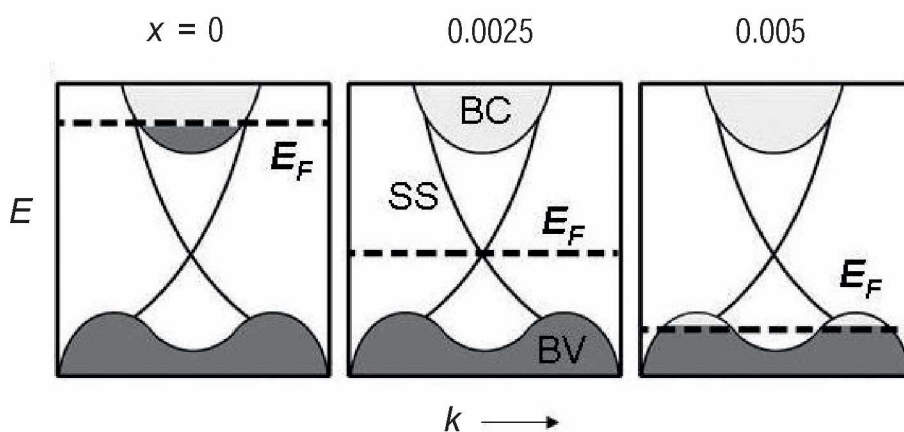
Rys. 3. Struktura pasmowa i przemieszczanie poziomu Fermiego w kryształach \text{Bi}_{2-x}\text{Ca}_x\text{Se}_3 przy x = 0, 0,0025, 0,005 ; BC – pasmo przewodnictwa, BV – pasmo walencyjne [5].
