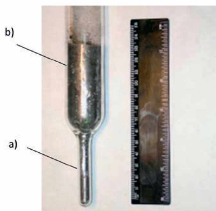
Rys. 5. Widok kryształu nr BS-8 w ampule po krystalizacji kierunkowej metodą VB i wygrzewaniu ujednorodniającym; a) - część zarodkowa; b) - część walcowa. Prędkość wzrostu \sim 3,5 mm/h, gradient temperatury w osi pieca G_0 = 15 °C/cm, temperaturę wygrzewania kryształu \sim 510 °C. Masa wsadu ok. 180 g.
