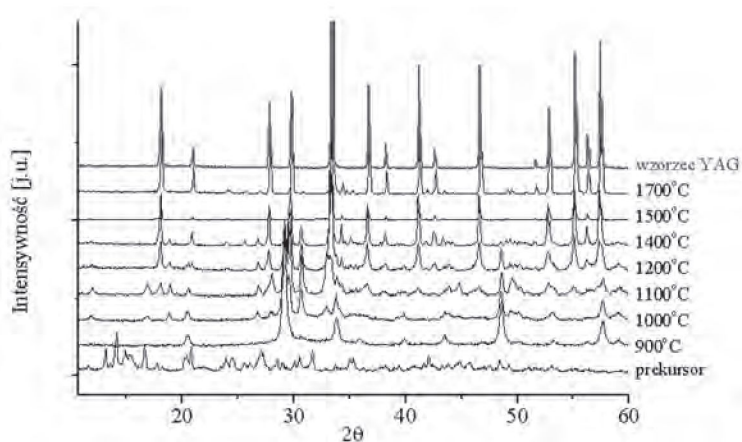
Rys. 5. Zestawienie dyfraktogramów proszku prekursora 0,2% Ce:YAG prażonego w powietrzu w zakresie 900°C-1700°C.
