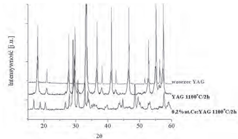
Rys. 8. Porównanie dyfraktogramów proszków YAG i 0,2% at. Ce:YAG prażonych w temperaturze 1100°C.
