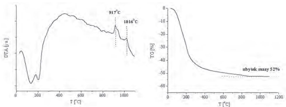
Rys. 3. Różnicowa analiza termiczna (DTA) i termogravimetria (TG) prekursora granatu itrowo-glinowego bez domieszki.
