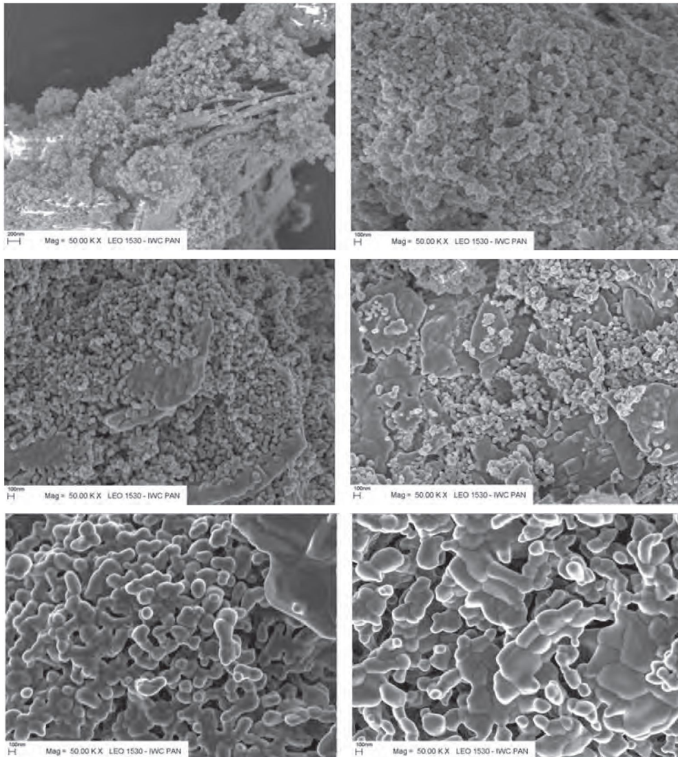
Rys. 10. Zdjęcia SEM nanoprozków 0,2% Ce:YAG i 2% Ce:YAG prażonych w 1000°C, 1200°C i 1400°C.
