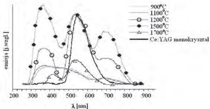
Rys. 13. Charakterystyki emisyjne proszków 2% Ce:YAG przy pobudzaniu długością fali 266 nm w zależności od temperatury syntezy. Fig. 13. Emission characteristics of 2% Ce:YAG powders excited at 266 nm.
