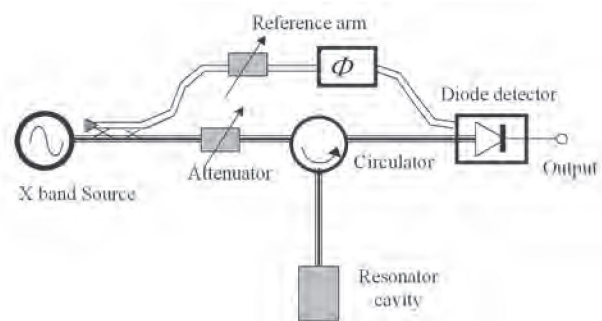
Fig. 2. Microwave signal path in EPR spectrometer. Rys. 2. Tor mikrofalowy w spektrometrze EPR.
