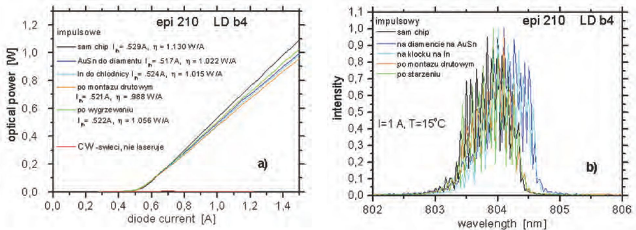
Rys. 5.1. Charakterystyki P-I i spektralne promieniowania laserowego dla DL z tak zwanym „zimnym” lutowaniem. Fig. 5.1. Light-current and spectral characteristics of LD with so-called „cold soldering”.
