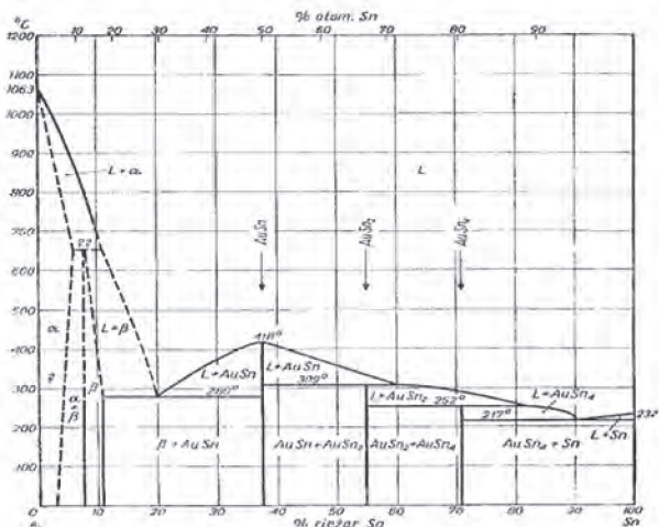
Rys. 3.1. Diagram fazowy Au-Sn. Fig. 3.1. Au-Sn phase diagram.
