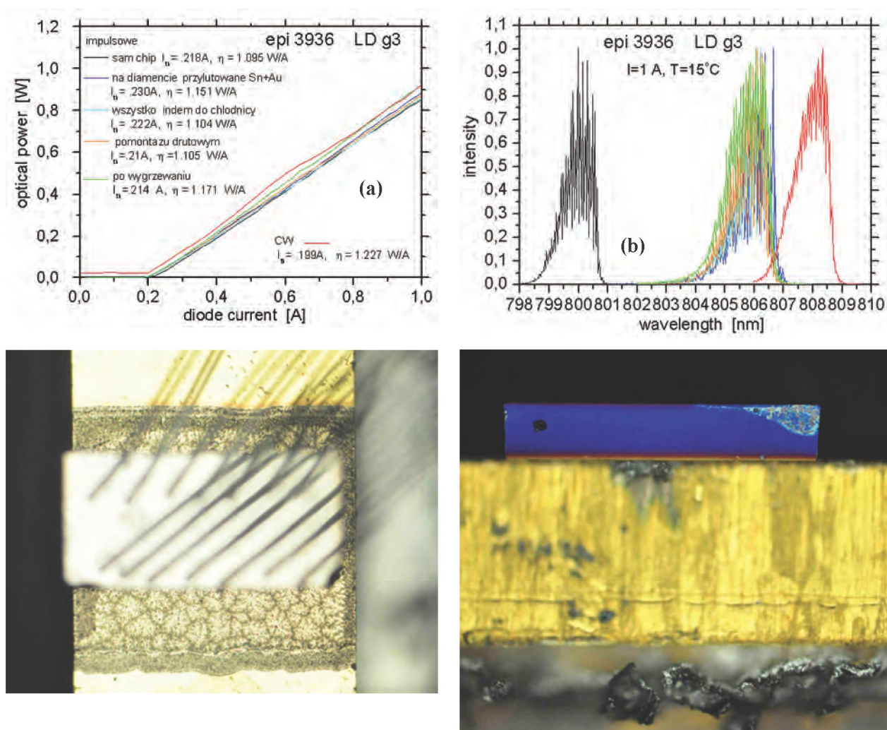
Rys. 4.2. Charakterystyki P-I (a) i spektralne (b) dla DL lutowanej przy pomocy napyłonych warstw Sn + 3,5 \mu\text{m} Au do diamentu i indem do chłodnicy Cu. Poniżej widok chipa z wyprowadzeniami drutowymi. Widoczna warstwa Sn+Au na diamentowej przekładce. Obok zdjęcie struktury od strony przedniego lustra.
