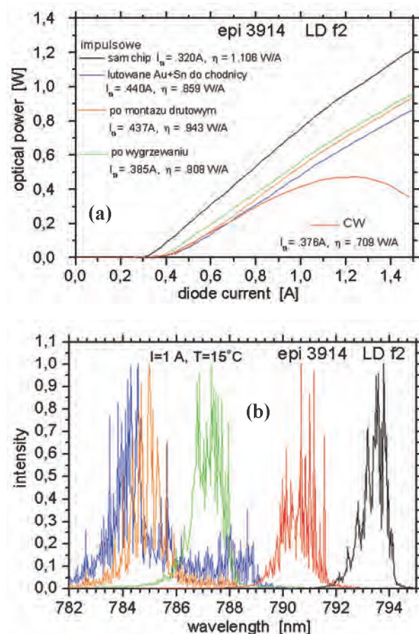
Rys. 3.6. Charakterystyki P-I (a) i spektralne (b) dla DL lutowanej do chłodnicy Cu przy pomocy napylnych warstw Sn + 3,5 \mu m Au.
