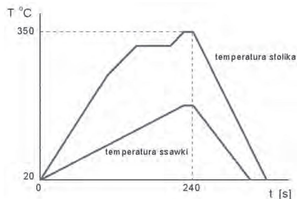
Rys. 3.2. Przykładowy przebieg temperatur w czasie lutowania chipu do chłodnicy przy użyciu folii AuSn Fig. 3.2. Exemplary temperature time-profile for a chip soldering onto a heat sink with AuSn perform foil.
