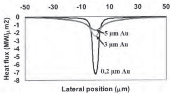
Rys. 1.1. Wpływ grubości warstwy Au osadzonej na stronie epitaksjalnej na rozprzestrzenienie strumienia ciepła emitowanego przez obszar aktywny diody laserowej. Punkt 0 jest środkiem obszaru aktywnego.
