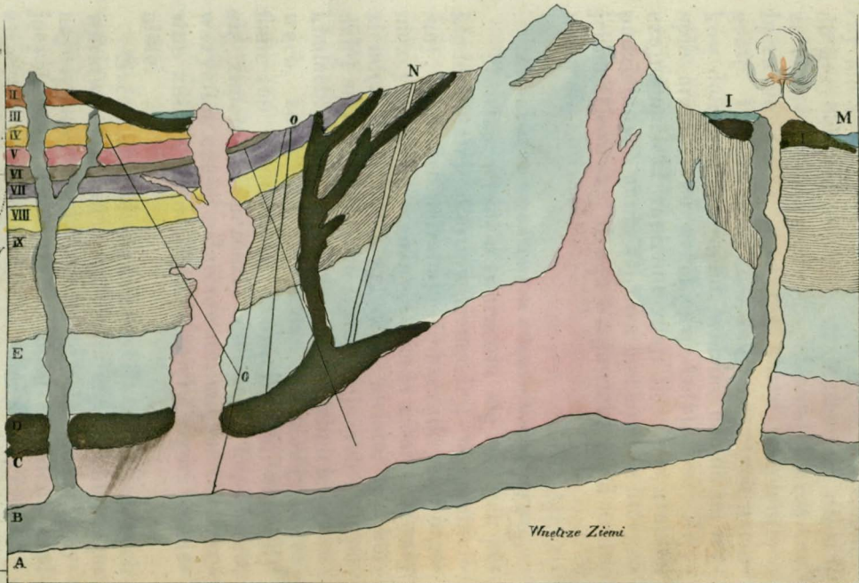
Obraz pokładów tworzących stałą powłokę Ziemi.
